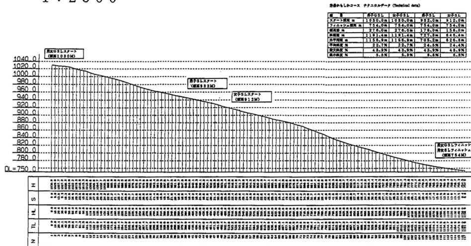
岩岳かもしかコース 縦断図 1 : 2500
