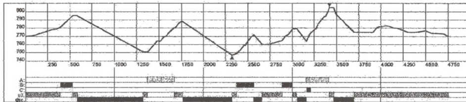
縦断面図
